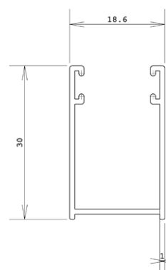
GUIDA - GUIDE
