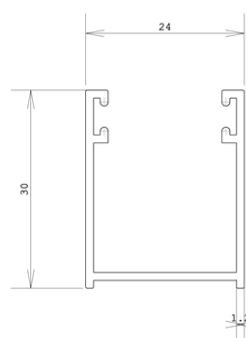
GUIDA - GUIDE
