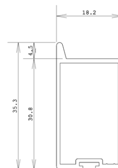
TRAVERSO - TRANSVERSE
